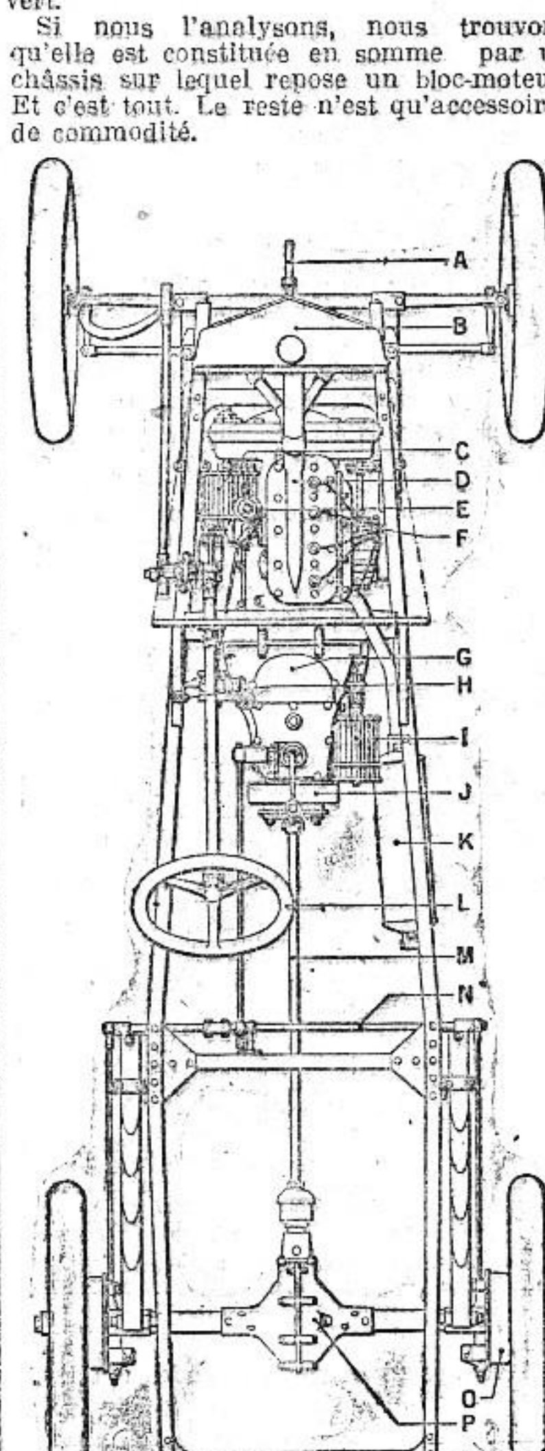
Ensemble du Châssis André CITROËN 1919
