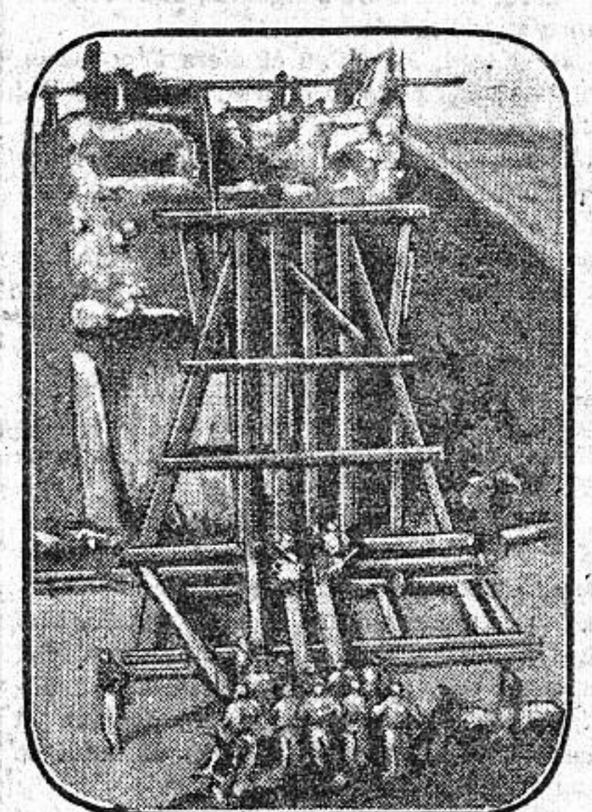
Construction de la pile intermédiaire
