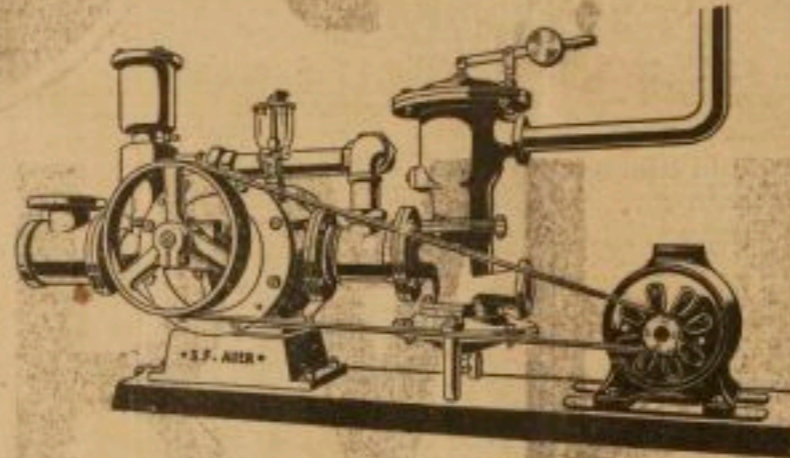
Mélangeur Compresseur "SFAGAZ" réglable, par le mélange préalable AIR et GAZ, la combustion intégrale du gaz. - ÉCONOMIE, SÉCURITÉ, RÉGULARITÉ, RAPIDITÉ, PROPRIÉTÉ. Primé au Concours de la Société Technique de l'Industrie du Gaz (Juin 1922).
