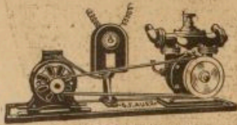
Élevateur de pression pour petites Industries (Bijouterie, Imprimerie, etc.) pouvant se brancher directement sur le Compteur Lumière.
